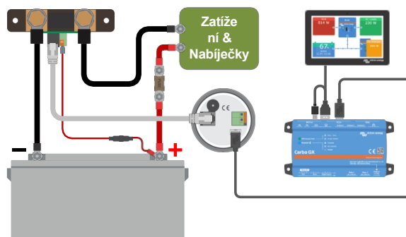
Monitor baterie je připojen k zařízení Cerbo GX a dotykové obrazovce GX.
